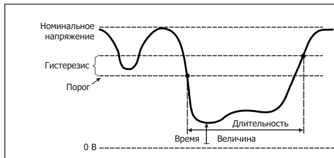
Рисунок 11. Характеристики прерывания напряжения
