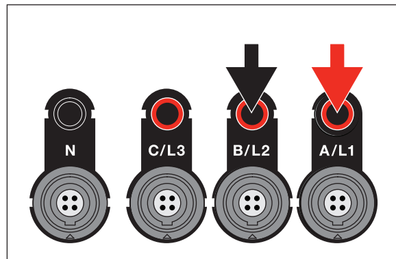
Рисунок 7. Сетевое напряжение без нейтрали
